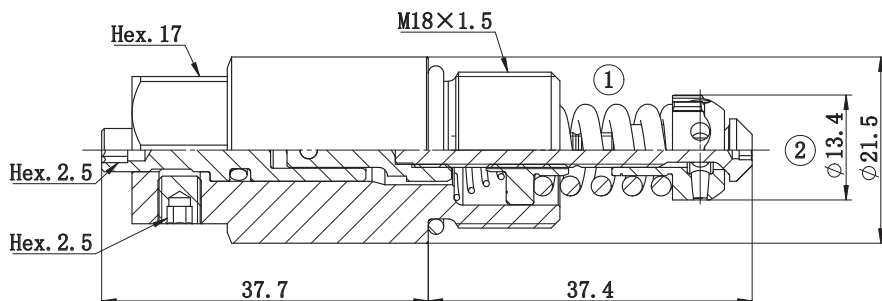
尺寸图 Dimensions
