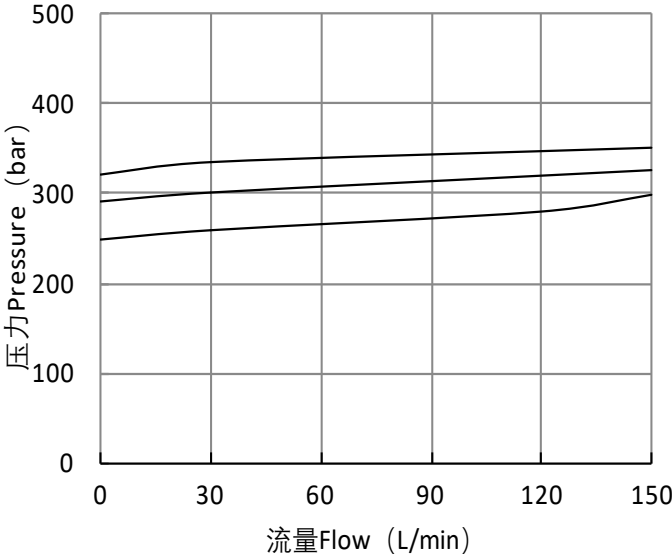
弹簧4=(251-320bar) Spring4= (251-320bar)
