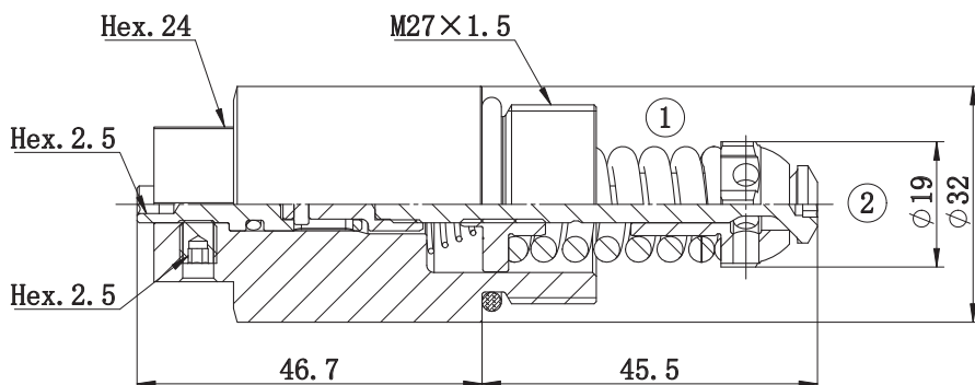
尺寸图 Dimensions
